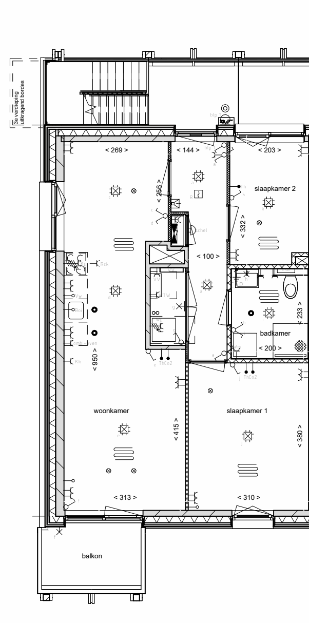
plattegrond
